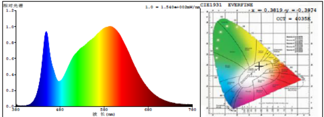
光谱分布
